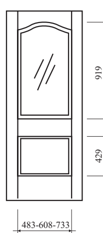
Modell SNB-3
