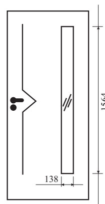
Modell V3LA
