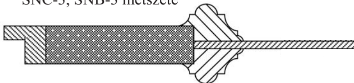
SNC-3, SNB-3 metszete
