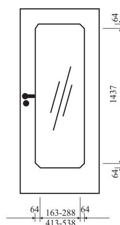
Modell H1LA
