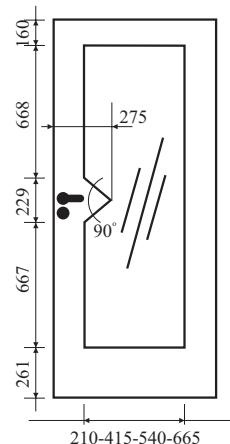
Modell V2LA
