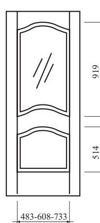
Modell SNC-3
